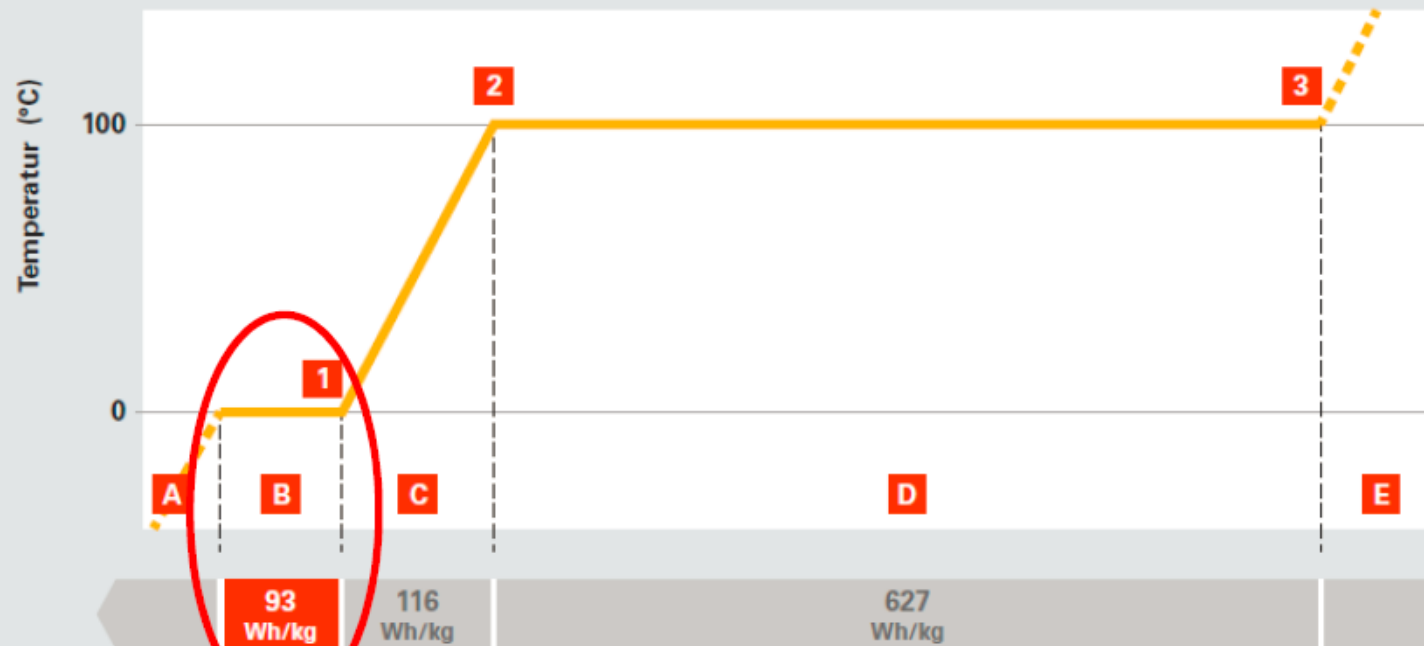
Abb. A.4.7-1 Wärmespeicher Phasenwechsel
